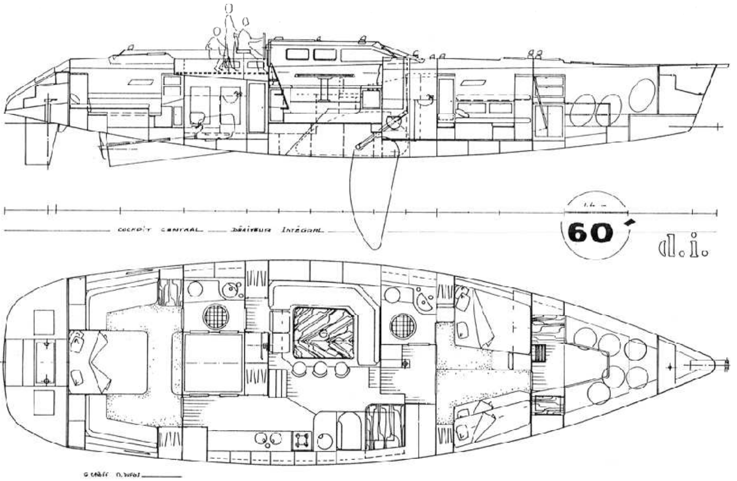
Salon de pont, cockpit central, cabine arrière.
