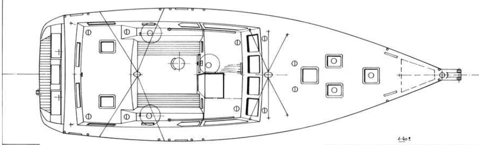
R.E. G. CARBÉ P. DUPUIS 43' SILHOUETTE ET DISPOSITION GÉNÉRALE DE PONT KETCH (ou cotre) A COCKPIT CENTRAL
