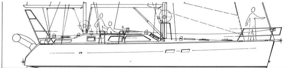
R.E. G. CARBÉ P. DUPUIS 43' SILHOUETTE ET DISPOSITION GÉNÉRALE DE PONT KETCH (ou cotre) A COCKPIT CENTRAL
